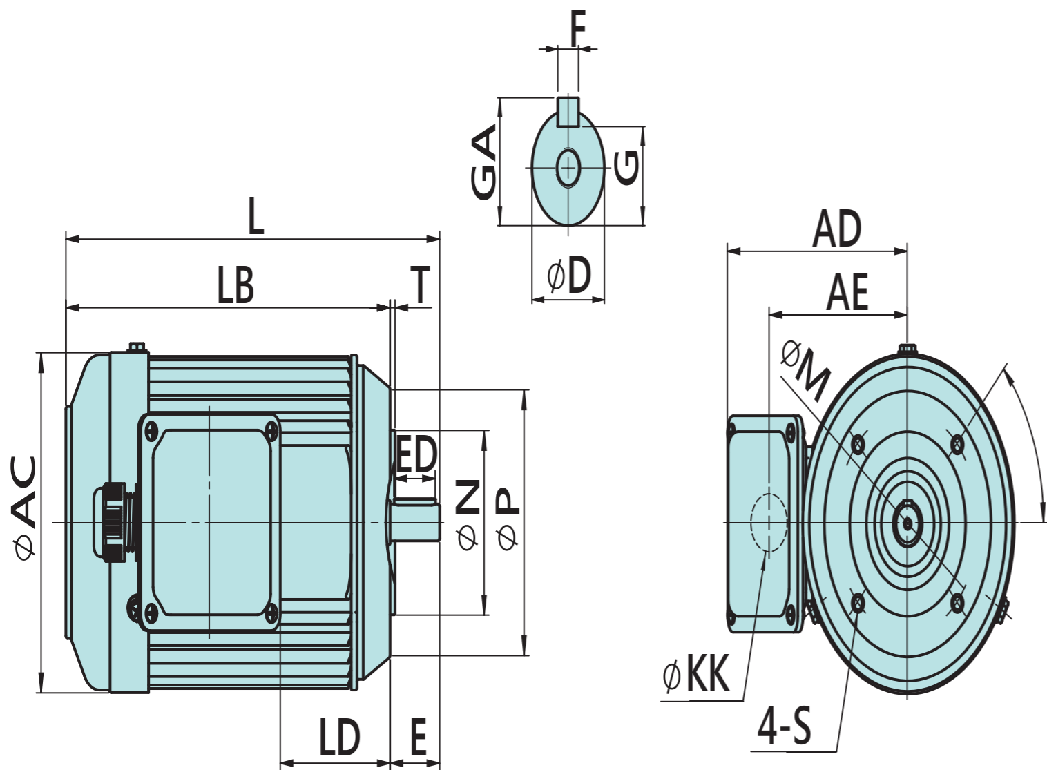
立式標準馬達 / CMVB 系列
