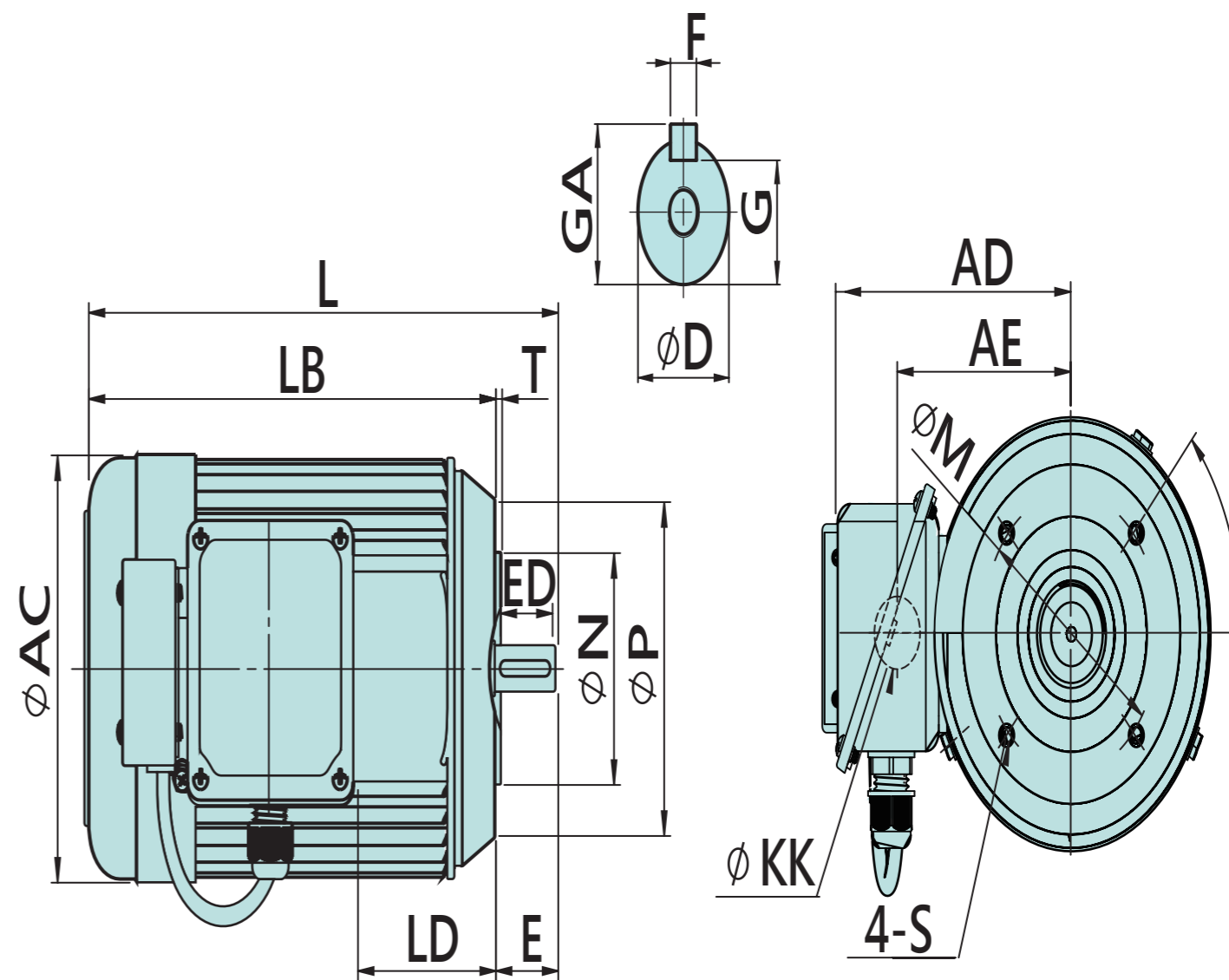
立式煞車馬達 / CMVBDA 系列
